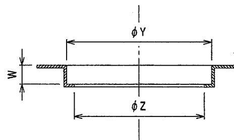
金属製流し台開口部寸法表
